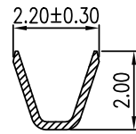
SEC A-A
