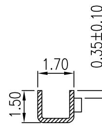
SEC D-D
